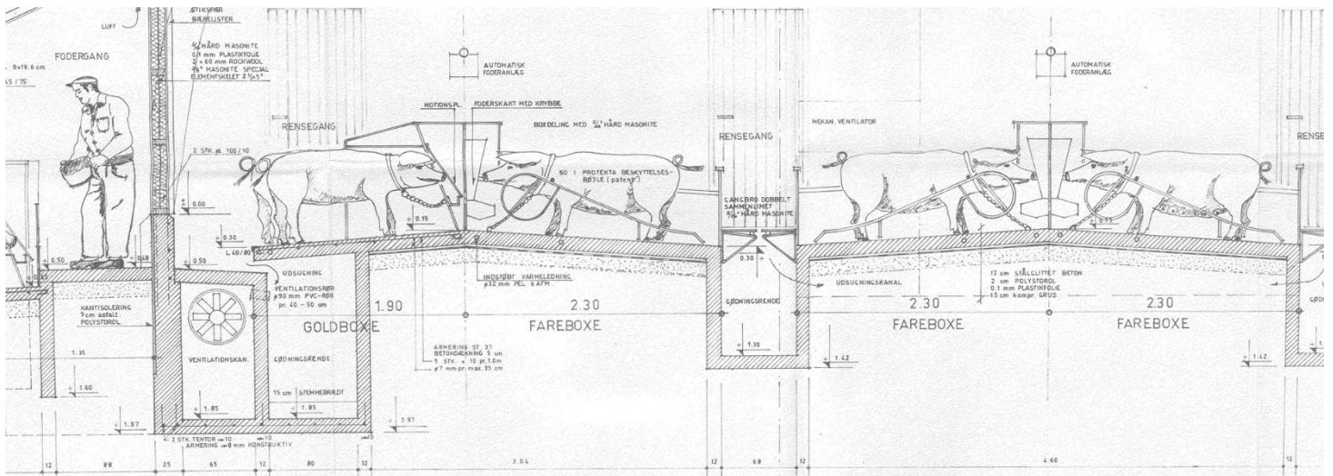
Original tværsnitstegning af Protekta sostald, ca. 1970.
